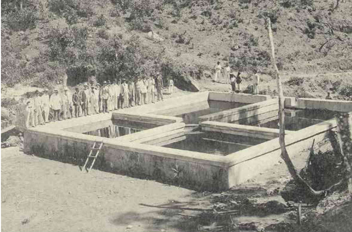
Tanques de filtração de água do rio Pau Amarelo, município de Cariacica (1912). APEES – Coleção Jerônimo Monteiro, 083.
